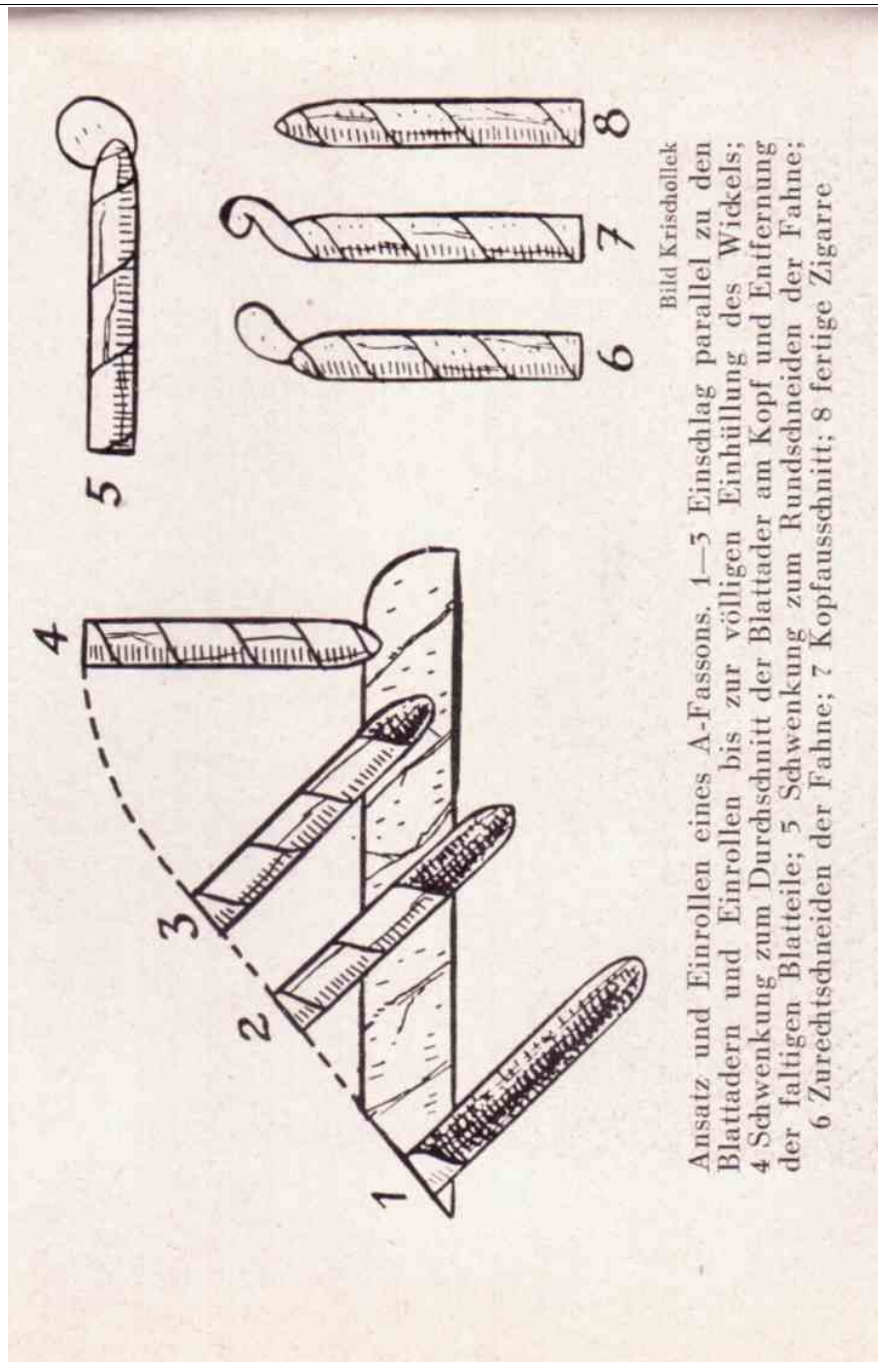
Bild 55: Rollen der Deckblätter mit „Schulter“: Die Blattrippen müssen parallel zur Zigarre liegen (aus Aschenbrenner/Stahl)
