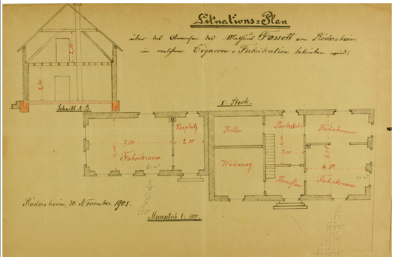
Bild 44: "Krankheit vorprogrammiert" - Plan der Fabrik "Fassott" in der Hauptstraße 214 aus dem Jahr 1905: der Wohnbereich ist minimal und umfasst alle Lebensbereiche: Schlafen, Essen, Wohnen. Die Toilette befindet sich außerhalb, die Flächen werden engräumig genutzt. Pro Personen genügen 2,5 m 2 Fläche - sei es zum Wohnen oder für den Arbeitsplatz.
